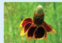
Mexican Hat
